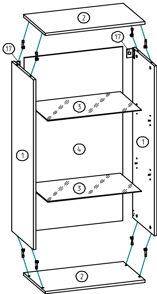
Схема сборки каркаса шкафа (рис.1)
