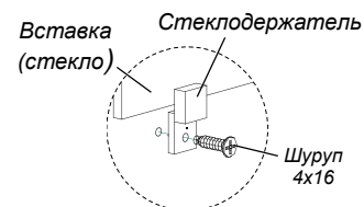
Схема крепления стеклодержателей (рис.5)
