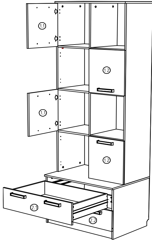
Схема навески фасадов (рис.1)
