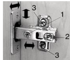
Схема регулировки четырёхшарнирной петли (рис.2)
