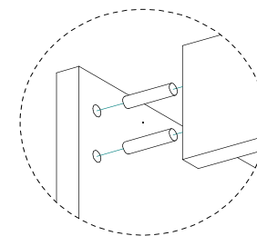
Схема установки шкантов (рис.6)
