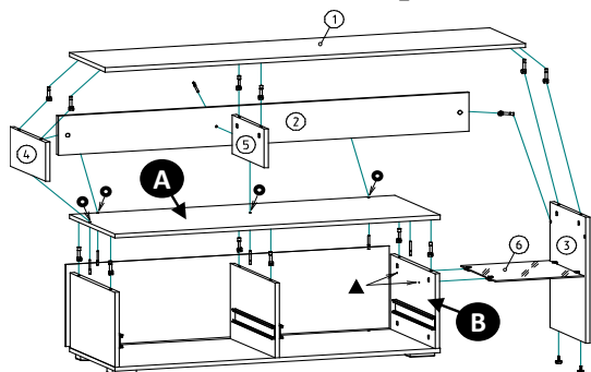
Схема сборки надстройки для тумбы ТВА (рис.1)
