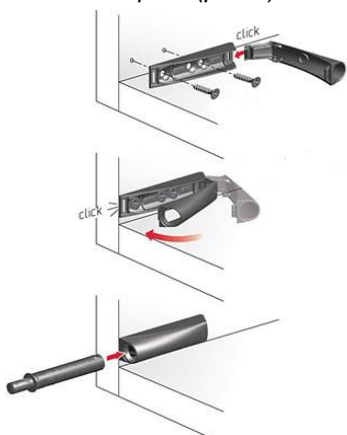
Схема установки толкателя (рис.10)
