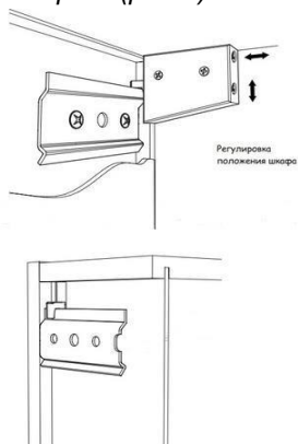
Схема регулирования подвески (рис.11)
