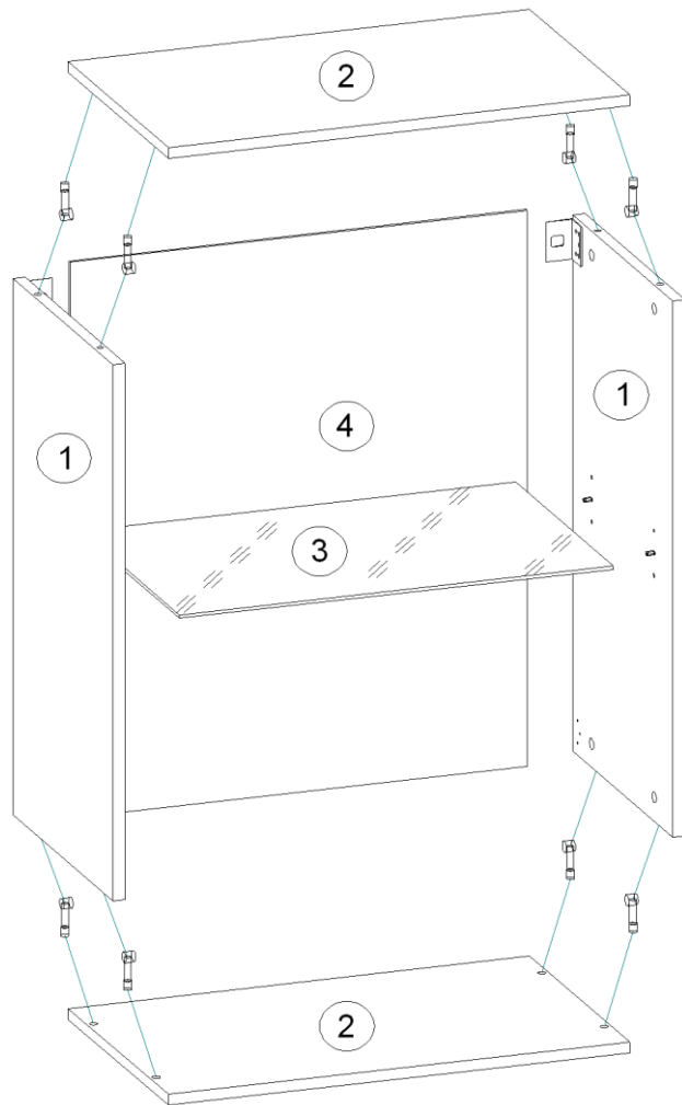
Схема сборки каркаса шкафа (рис.1)
